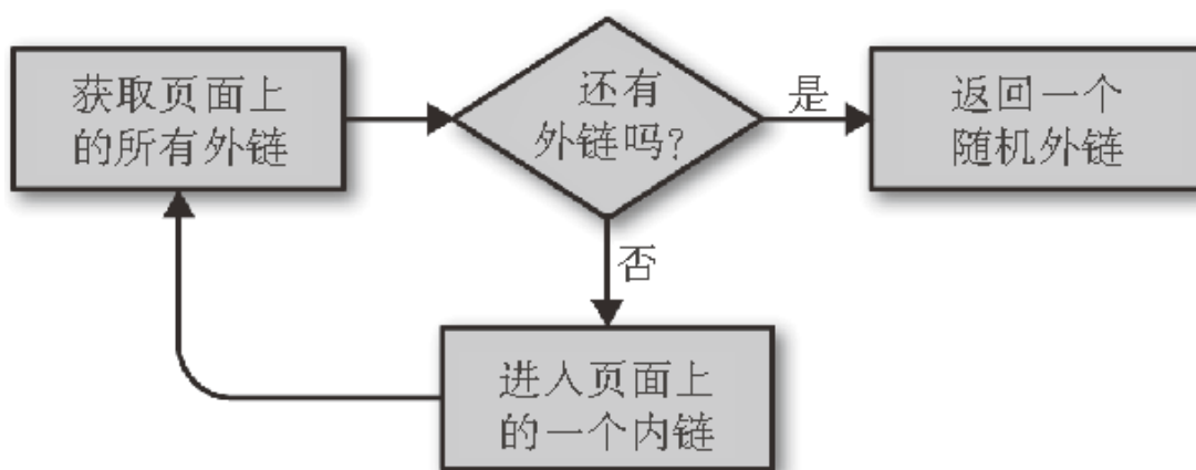
图 3-1：从互联网上不同的网站采集外链的程序流程图
