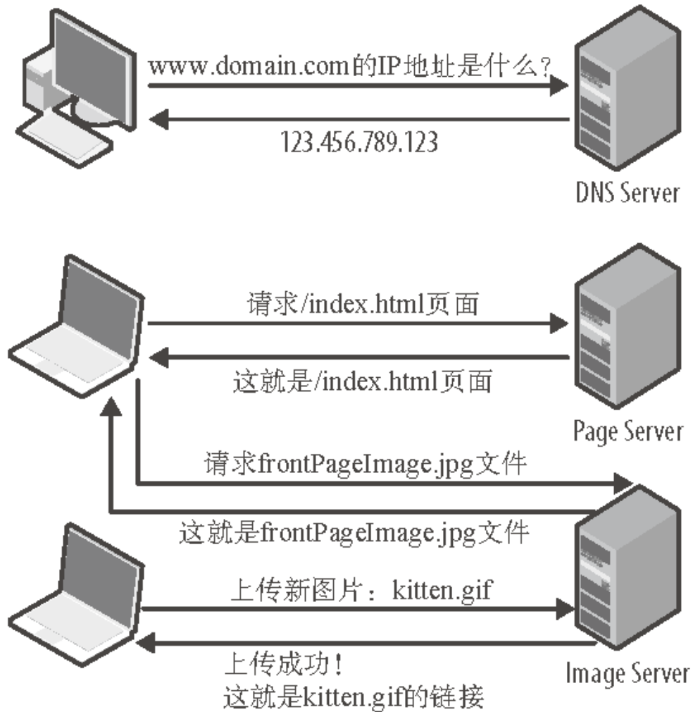
图 B-1：若干常见客户端 - 服务器互联网模型数据交换方式
