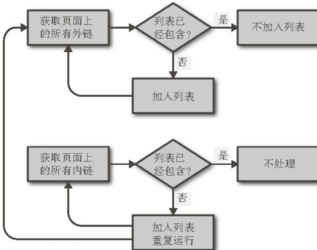
图 3-2：收集内链和外链的程序流程图
