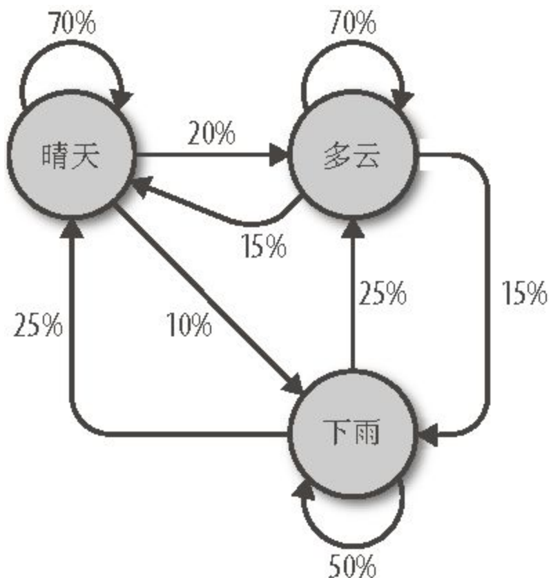
图 8-1：马尔可夫模型描述的理论天气系统
