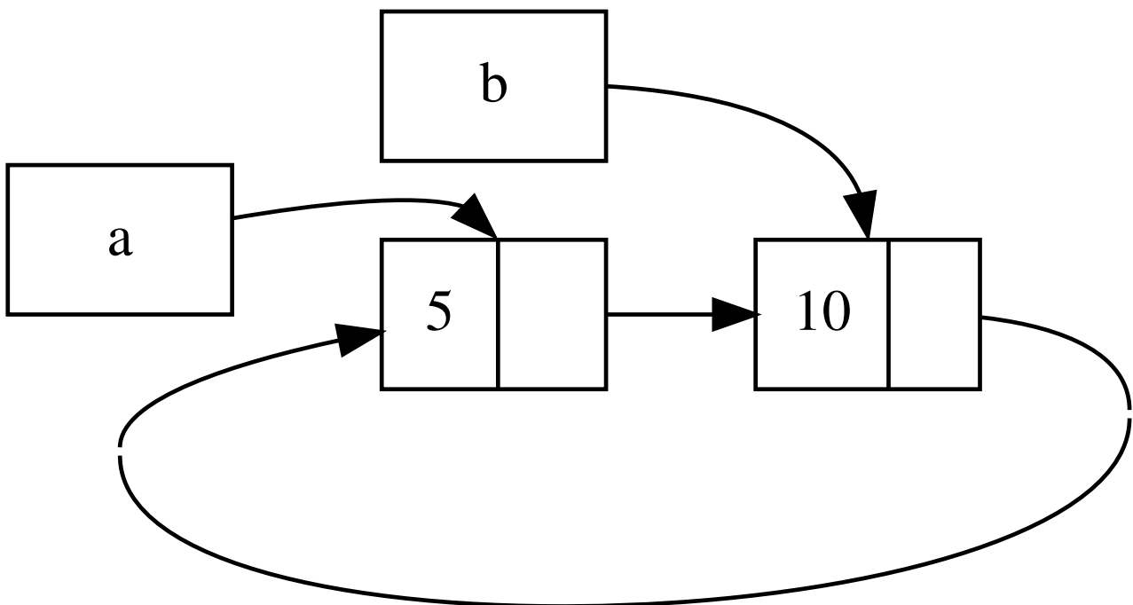
图 15-4: 列表 a 和 b 彼此互相指向形成引用循环
