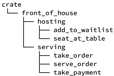
示例 7-2: 示例 7-1 中代码的模块树
