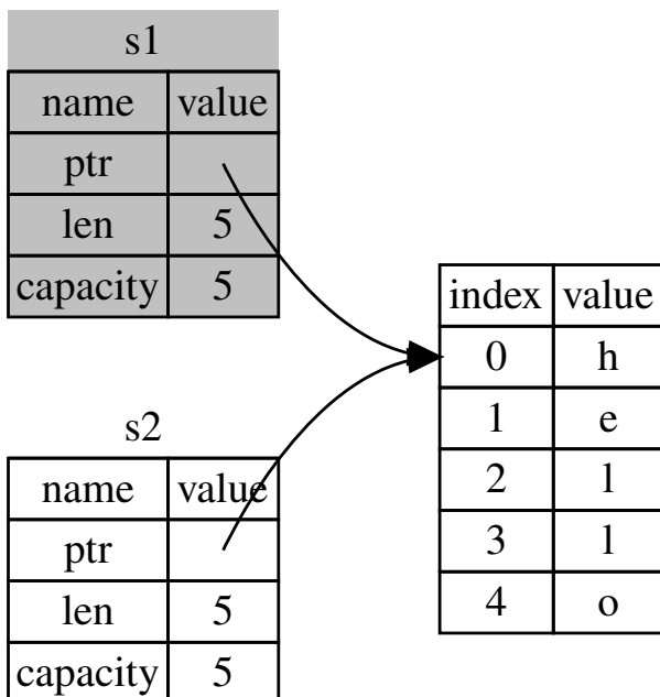
图 4-4: s1 无效之后的内存表现
